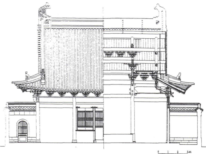
上海真如寺正殿从断面及立面图
