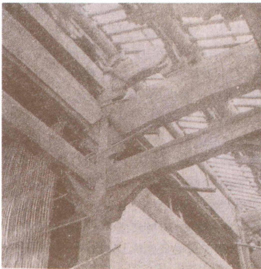
图二 后槽乳枋、栌斗及随梁
