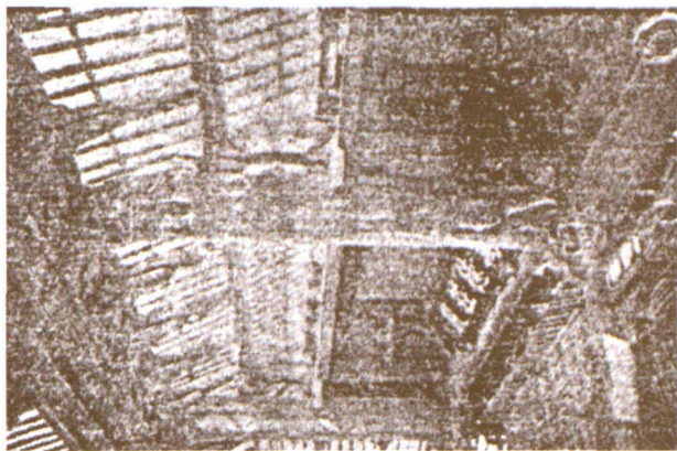
图一 前槽轩大梁东乙、东式,蜀柱、上步梁及轩平基、轩平基斗拱,外檐斗拱后尾
