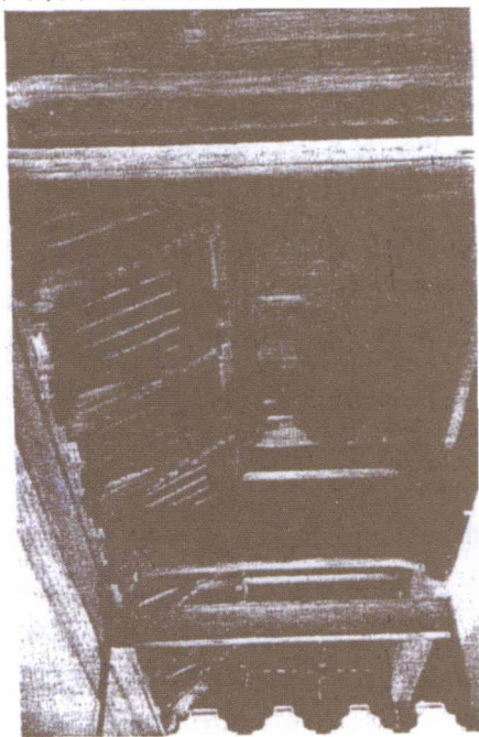
上海真如寺正殿从横梁结构之一
