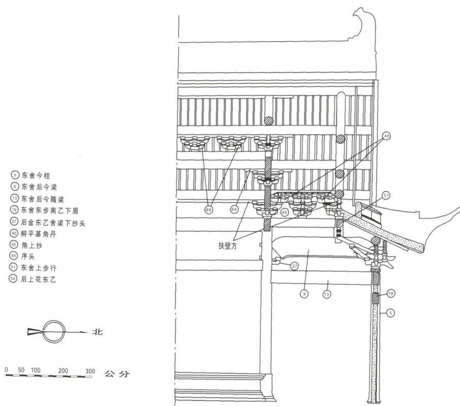
图六 真如寺构件部位名称图
