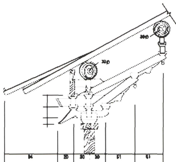
图九 真如寺外檐斗拱
