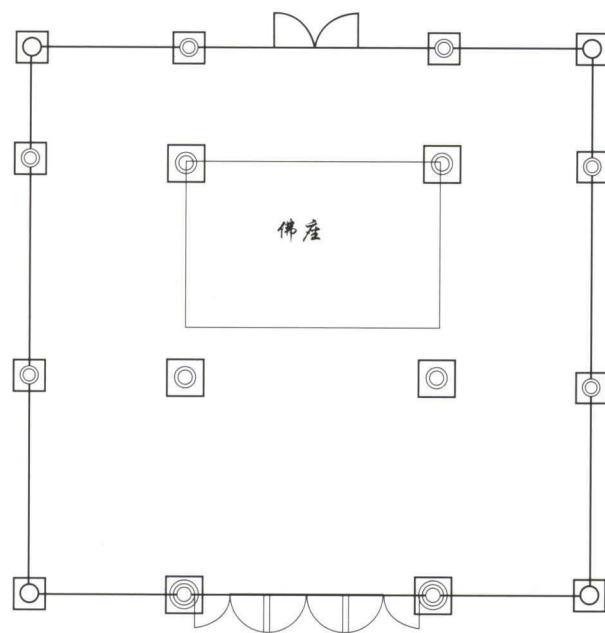
图八 真如寺柱础平面图
