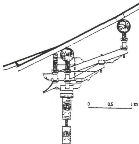
上海真如寺正殿柱头铺作
