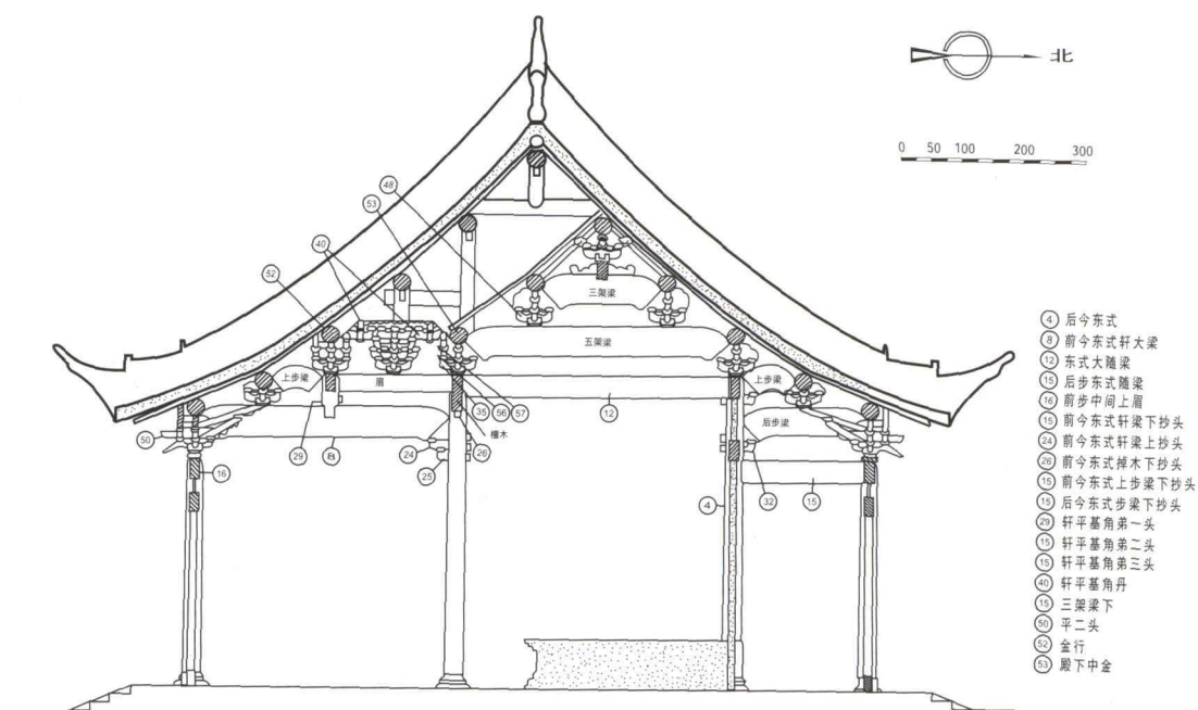
图五 真如寺构件部位名称图
