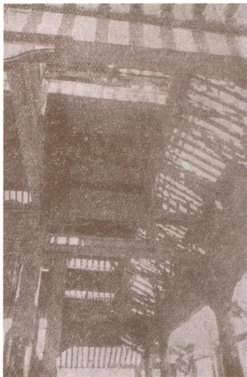
图三 东次间乳枋、蜀柱、随梁枋及三架椽长之素枋
