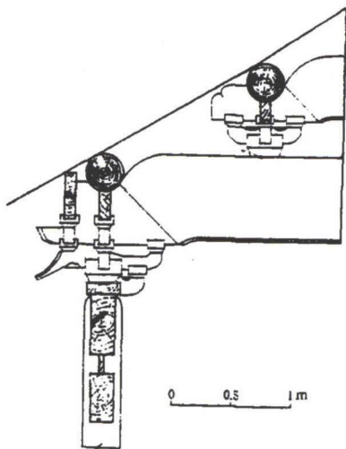
上海真如寺正殿补间铺作
