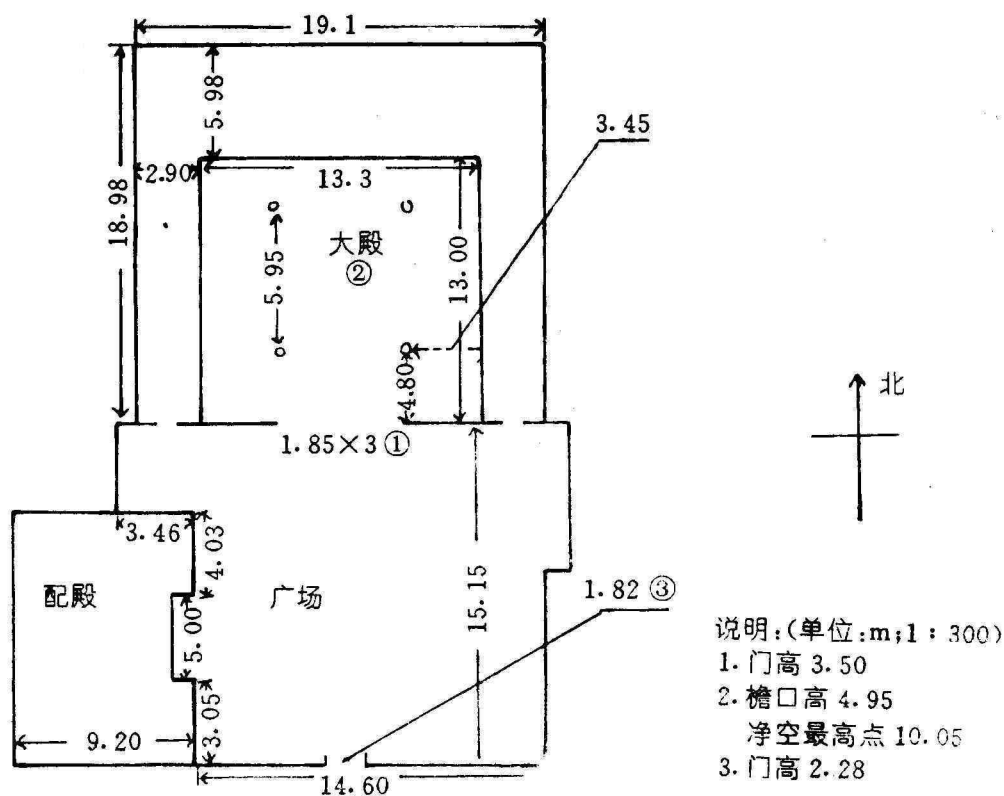
真如寺大殿平面图
