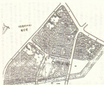
甘泉新村北块规划示意图
